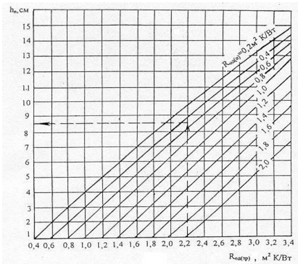
Рисунок 2.1 - График для определения требуемой толщины теплоизолирующего слоя из пенополистирольных плит «ТЕХНОПЛЕКС».
