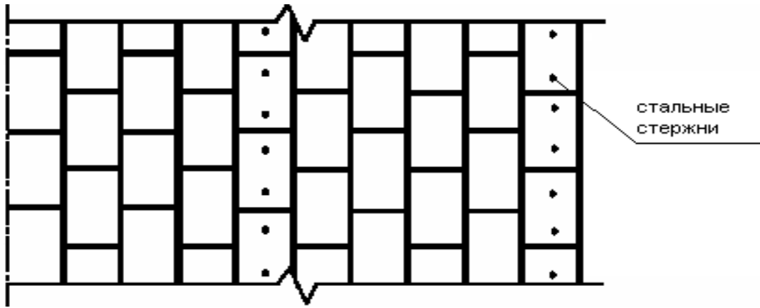
Рисунок 4.1 - Схема раскладки плит «ТЕХНОПЛЕКС»
